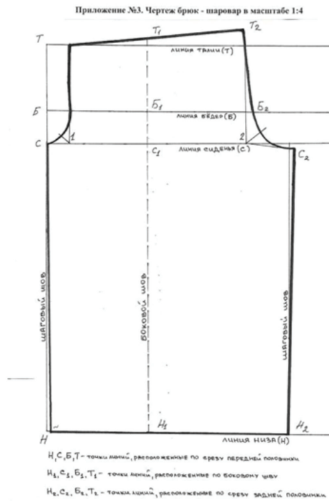
Чертеж брюк-шаровар в масштабе 1:4
